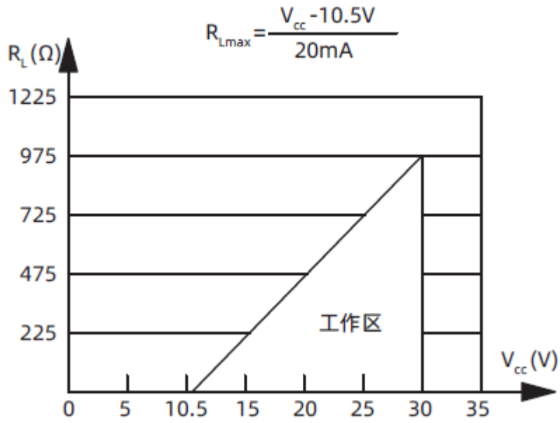
图 2 负载特性图
