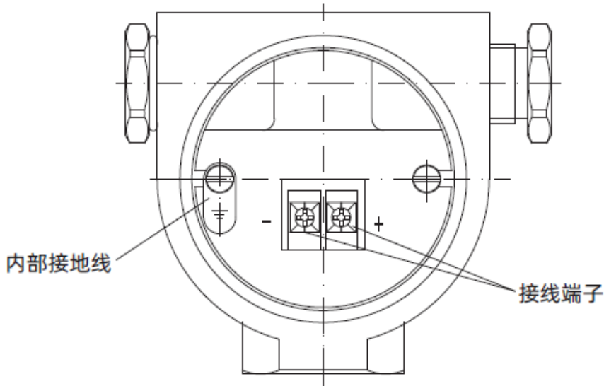
图 6 远传接线图
