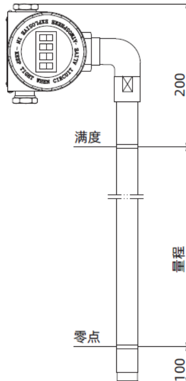
图 3 远传装置
